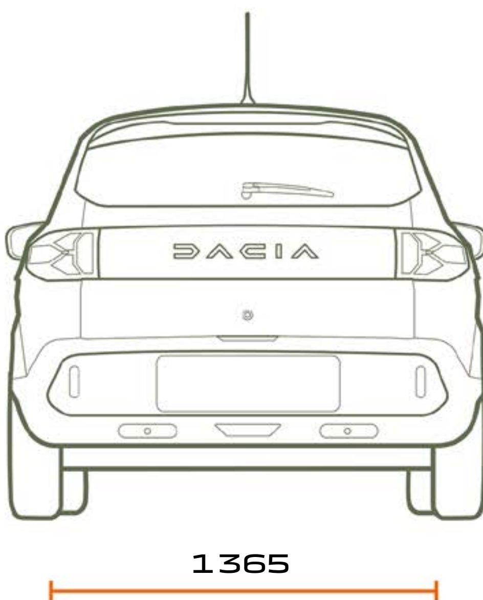
VUE ARRIÈRE
